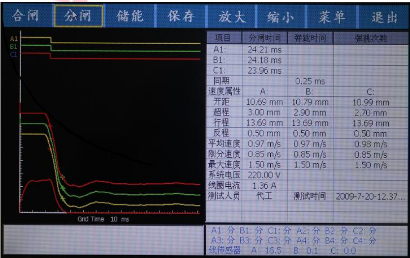
5、3 路传感器分闸测试数据如下图:
