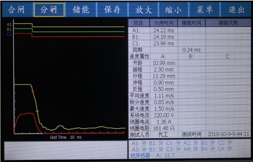
4、3 路传感器合闸测试数据如下图:
