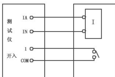
单相反时限接线
