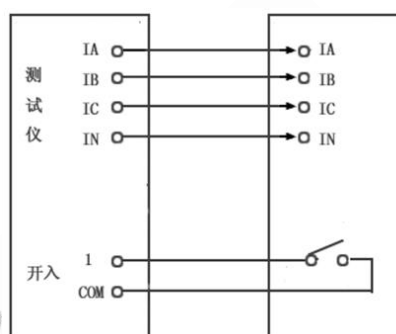
三相反时限接线
