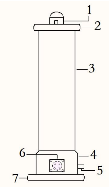
图 1.2 倍压筒结构图
